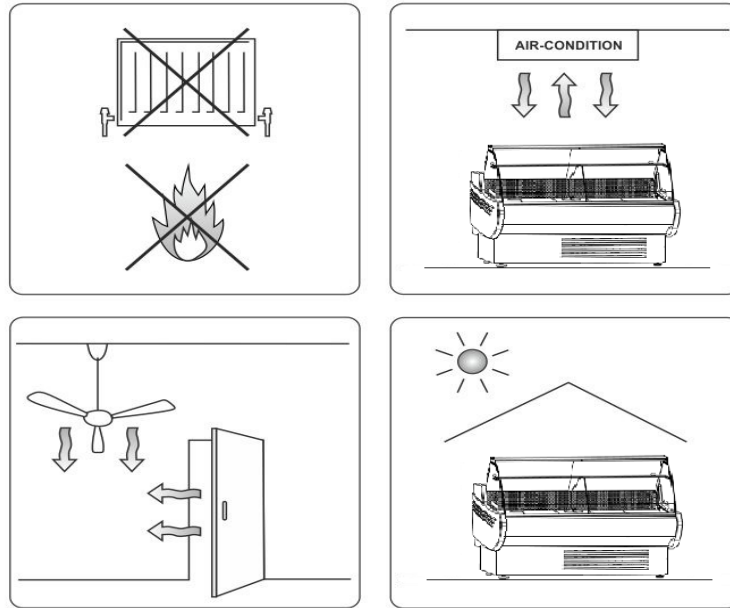
Рисунок 3 – Розміщення вітрини
