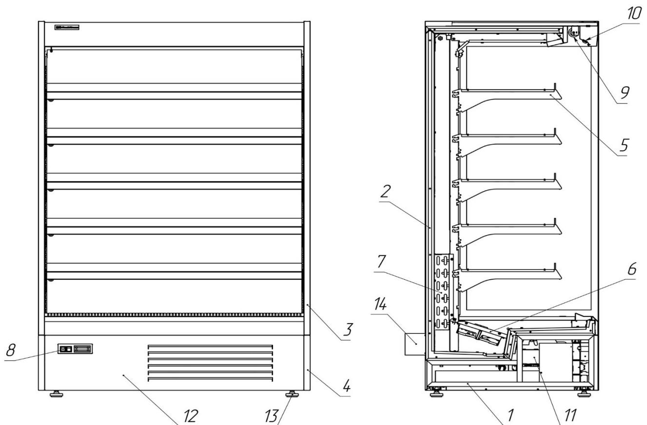
Рисунок 2 – Размещение основных узлов и комплектующих
